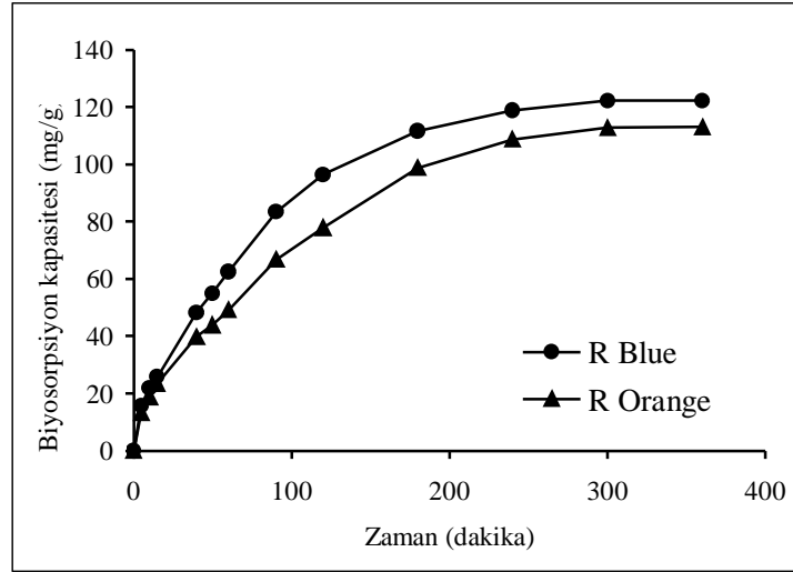
Şekil 4.8. Asit ile işlem gören biyokütle ile R Blue ve R Orange biyosorpsiyonunun zamana bağlılığı (başlangıç boya konsantrasyonu, 100mg/L)
