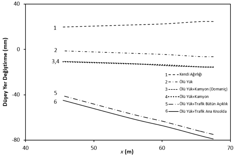
Şekil 24. Yüklemelere karşı gelen yerdeğiştirmeler
