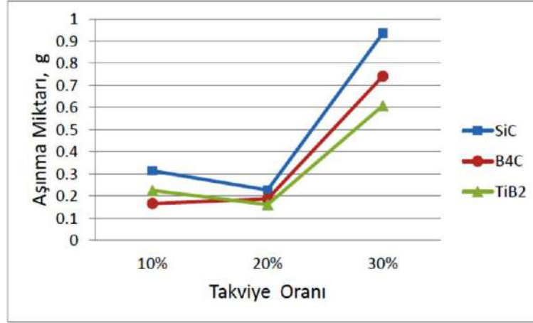
Şekil 9. Kompozit numunelere ait aşınma miktarı değerleri
