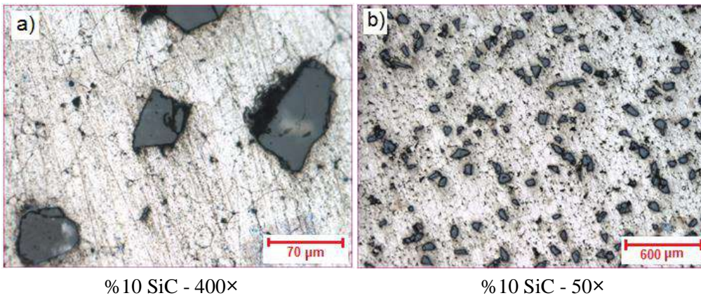
Şekil 3. SiC takviyeli AA7075 kompozitlerin optik mikroskop görüntüleri
