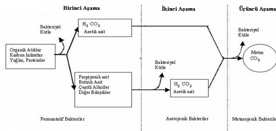
Şekil 1: Biyogaz üretim aşamaları (25).
