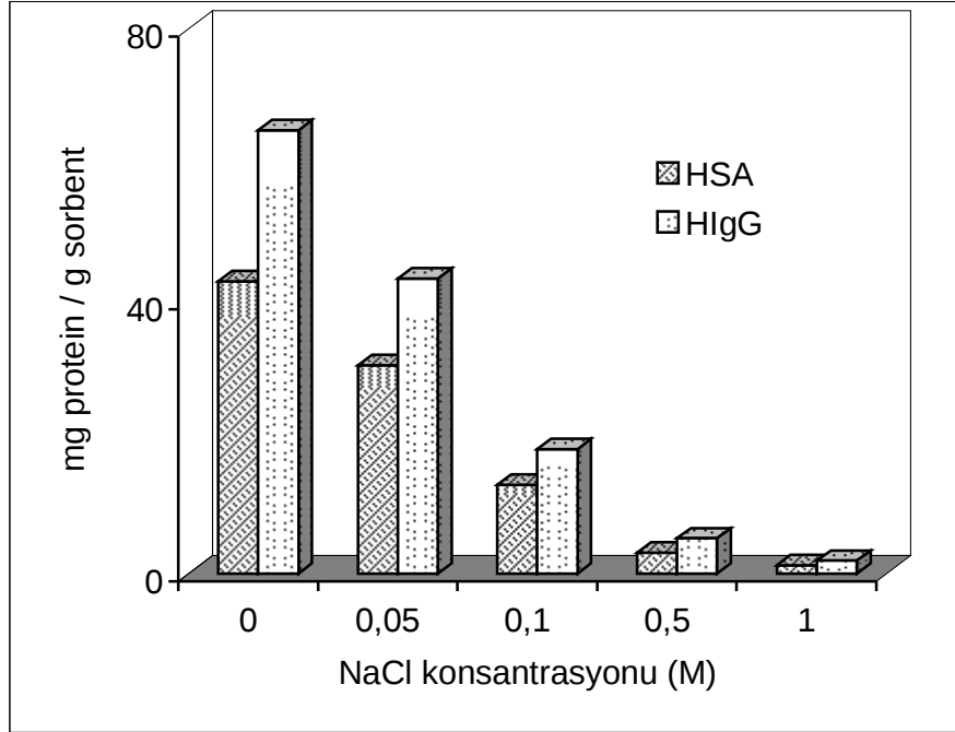
Şekil 4.10. Afinite hidrojel ile sulu ortamdan protein adsorpsiyonuna iyonik şiddetin etkisi
