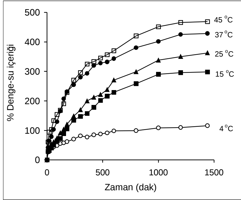
Şekil 4.2. Partikül yapıdaki p(AAc-AA) afinite hidrojenlerinin farklı sıcaklıklardaki denge su içeriği davranışı
