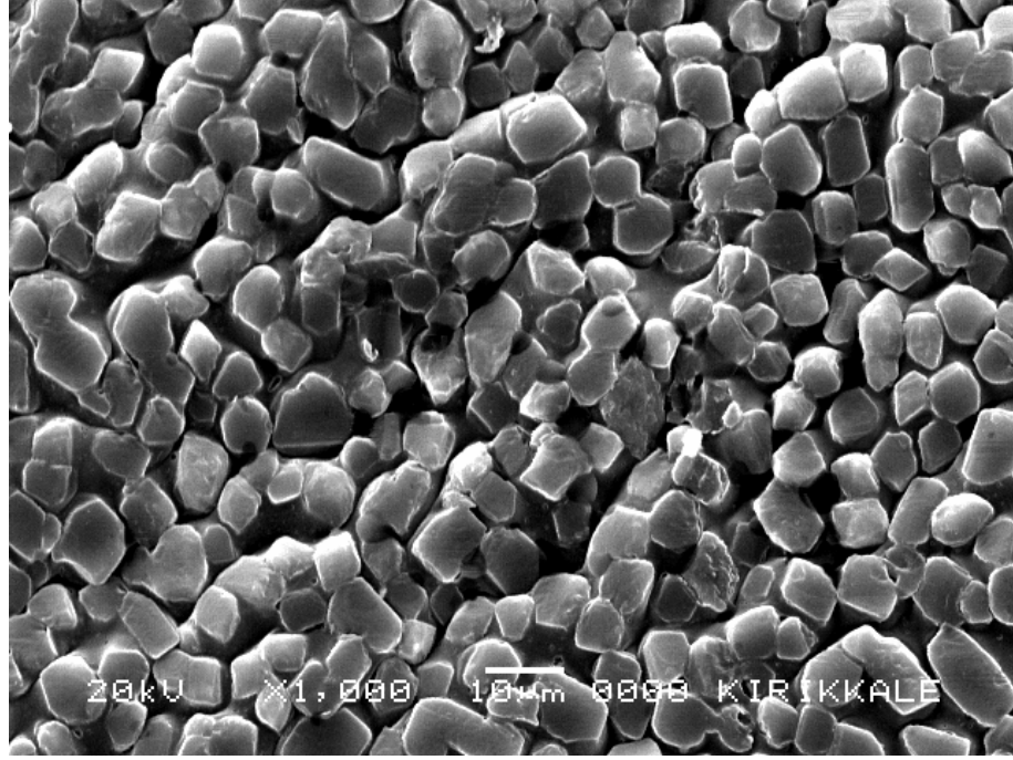
Şekil 4.3. Partikül yapıdaki p(AAc-AA) afinite hidrojelinin SEM mikrografı
