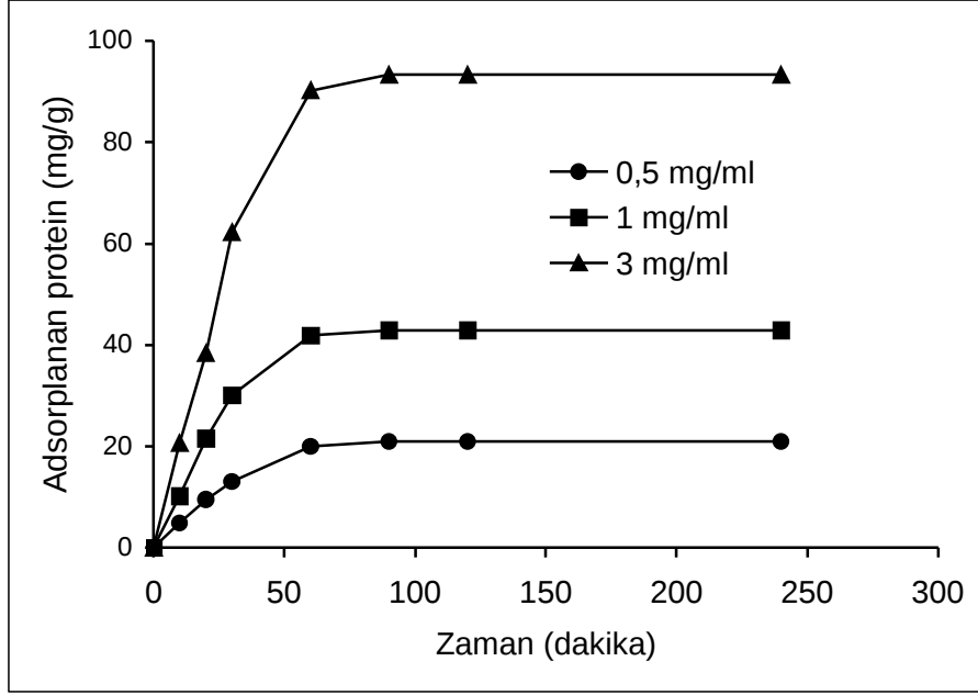
řekil 4.7. p(AAc-AA) afinite hidrojele HSA adsorpsiyonunda denge zamanı
