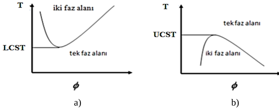
Şekil 3.17. Sıcaklık duyarlı polimerlerin faz diyagramları [65].
