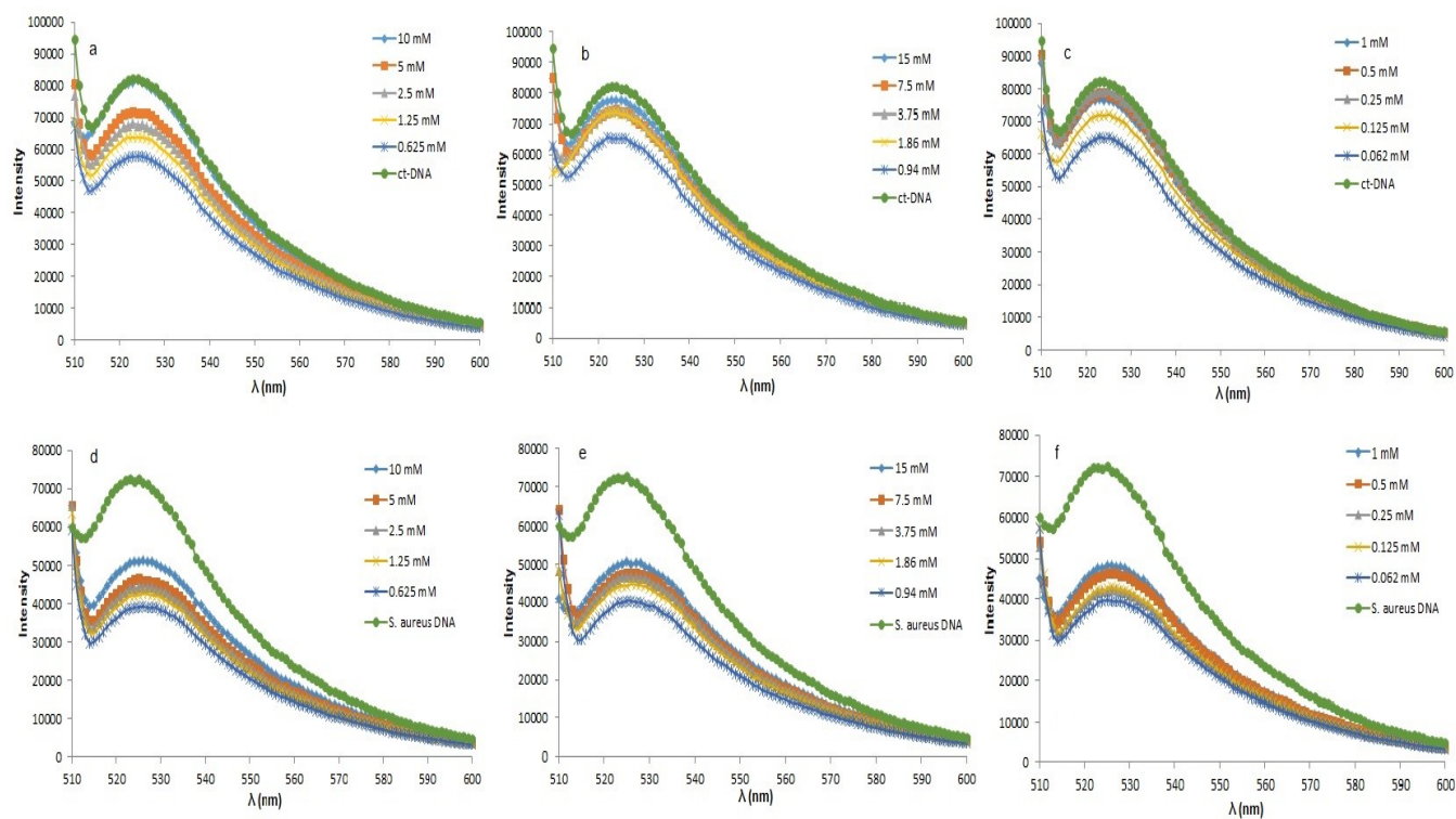
Fig. 3 – Fluorescence spectra of genomic DNA+melamine/metabolites. (a) ct-DNA+melamine, (b) ct-DNA+cyanuric acid, (c) ct-DNA+uric acid, (d) S. aureus DNA+melamine, (e) S. aureus DNA+cyanuric acid, (f) S. aureus DNA+uric acid.
