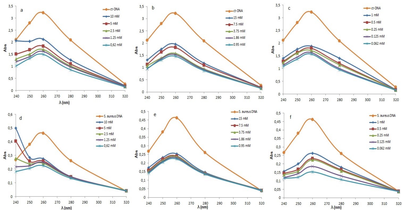
Fig. 2 – UV-absorbance spectra of genomic DNA+melamine/metabolites. (a) ct-DNA+melamine, (b) ct-DNA+cyanuric acid, (c) ct-DNA+uric acid, (d) S. aureus DNA+melamine, (e) S. aureus DNA+cyanuric acid, and (f) S. aureus DNA+uric acid.
