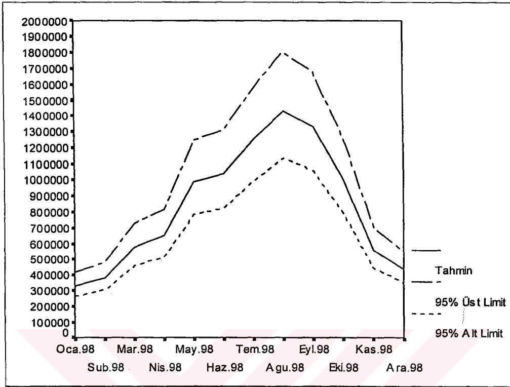
Şekil-6.14. Son Bir Yıla Ait Aylık Turist Sayısı Tahminleri ile Alt-Üst Sınır Değerlerinin Grafiği
