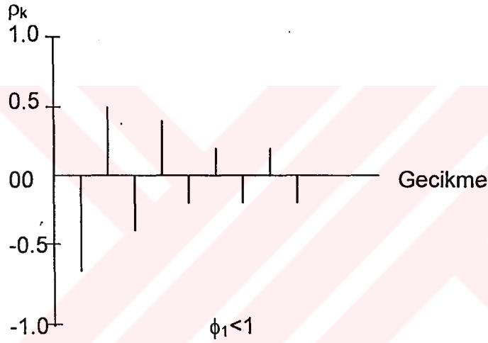
Şekil-3.2. Birinci Mertebeden Otoregresif Sürecin \phi_1 'e Bağlı Otokorelasyon Fonksiyonu
