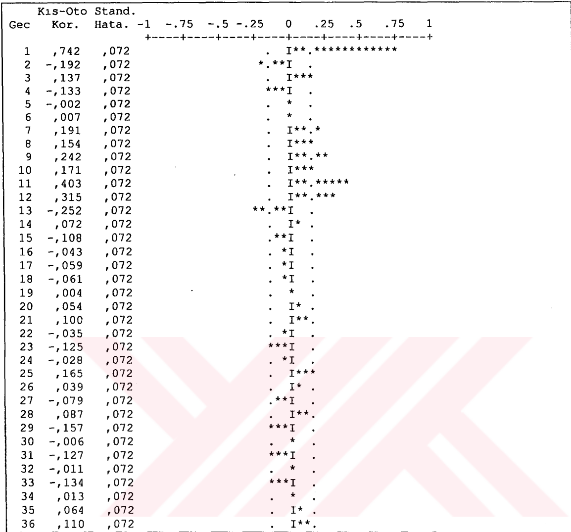
Şekil-6.6. Türkiye'nin.Turizm Geliri Serisinin Kısmi Otokorelasyon Grafiği
