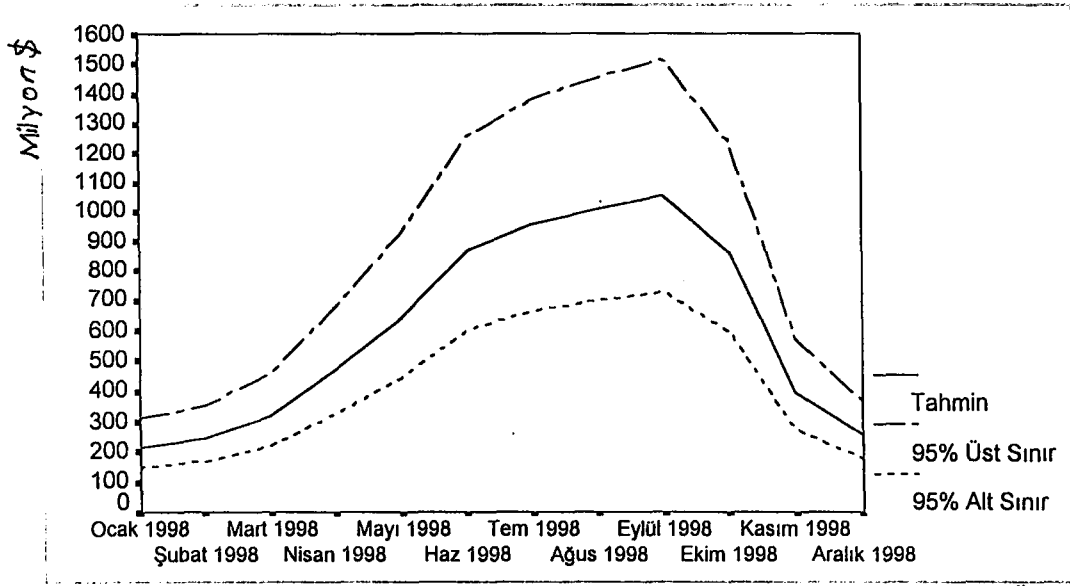
Şekil-6.19. Son Bir Yıla Ait Aylık Turizm Geliri Tahminleri ile Alt-Üst Sınır Değerlerinin Grafiği
