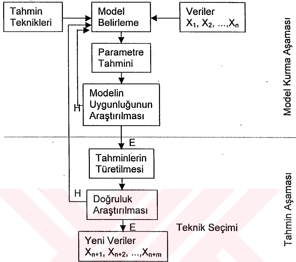
Şekil-1.1. Sayısal Tahmin Sürecinin Aşamaları
