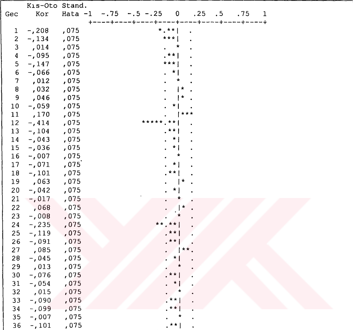
Şekil-6.12. Durağanlaştırılmış Turizm Geliri Serisinin Kısmi Otokorelasyon Grafiği
