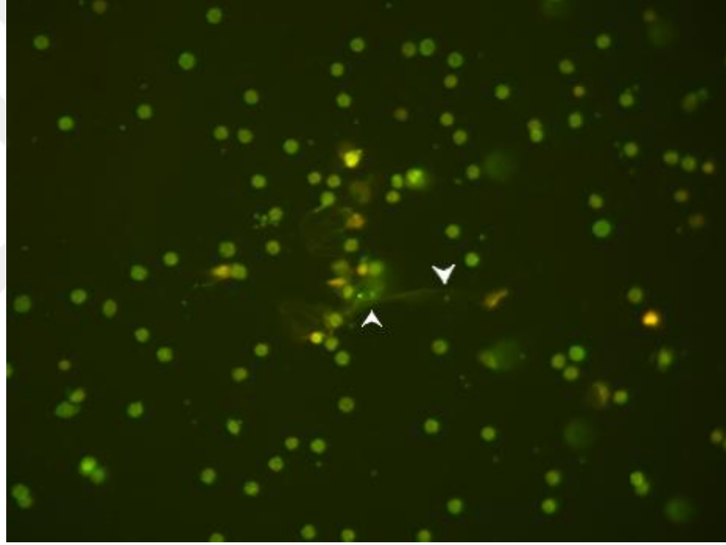
Şekil 3.3. Toxoplasma gondii tachyzoitlerine karşı köpek PMN'inde gelişen hücre dışı tuzaklardaki histon (H3)'u gösteren floresans mikrograf (Oklar: Hücre dışı tuzaklar arasındaki tachyzoitler).
