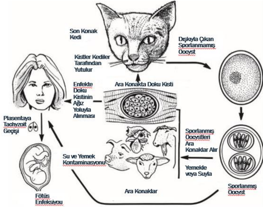
Şekil 1.3. Toxoplasma gondii 'nin yaşam çemberi (Dubey 2010).
