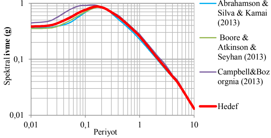
Şekil 5. Azalım ilişkilerine göre hedef spektrum için spektral ivme-periyot grafiği (Spectral acceleration-period graph for the target spectrum with respect to attenuation relationships)
