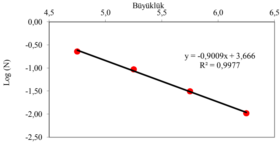
Şekil 6. Deprem büyüklüğü-oluşum sayısı ilişkisi (Earthquake magnitude- number of occurrence relationship)
