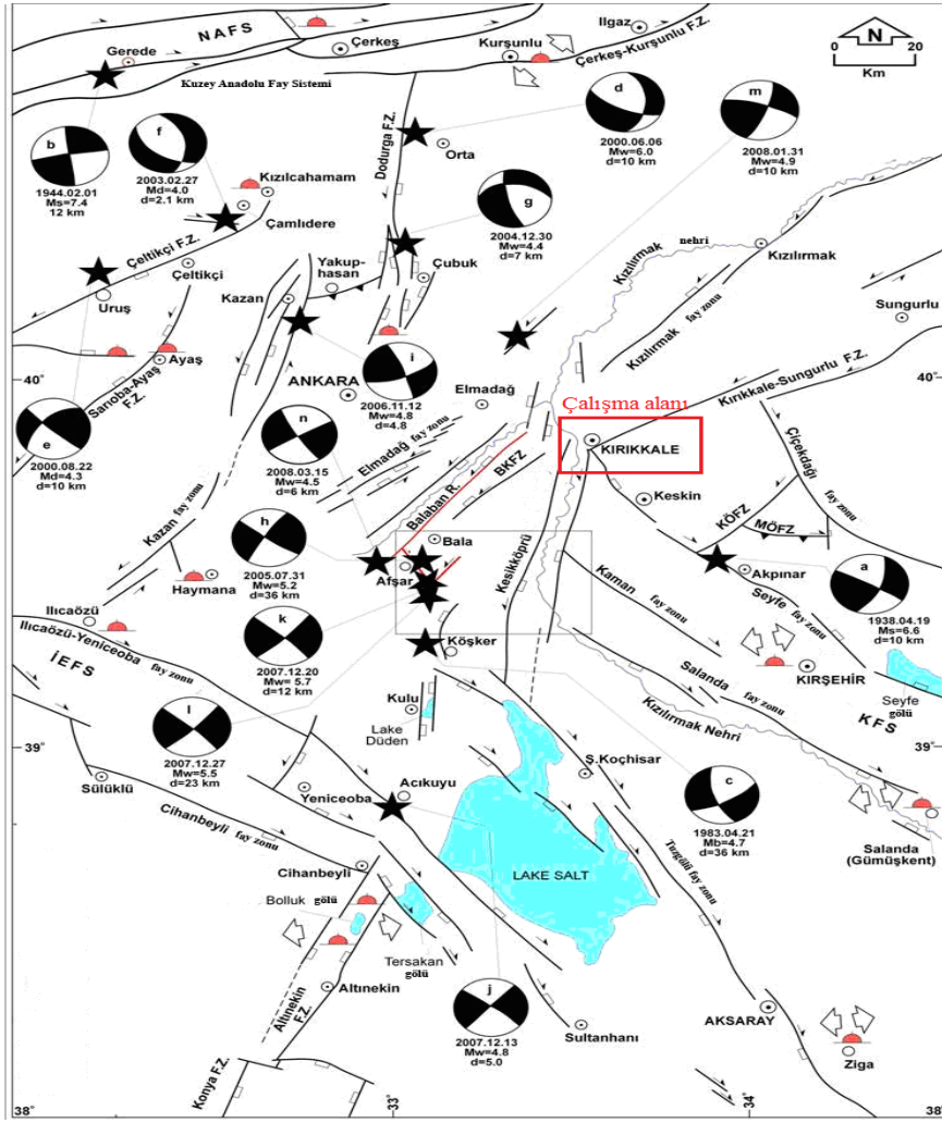
Şekil 3. Kırıkkale etrafındaki önemli depremlerin merkez üssü dağılımı (The distribution of the epicenters of major earthquake around Kırıkkale) [14]
