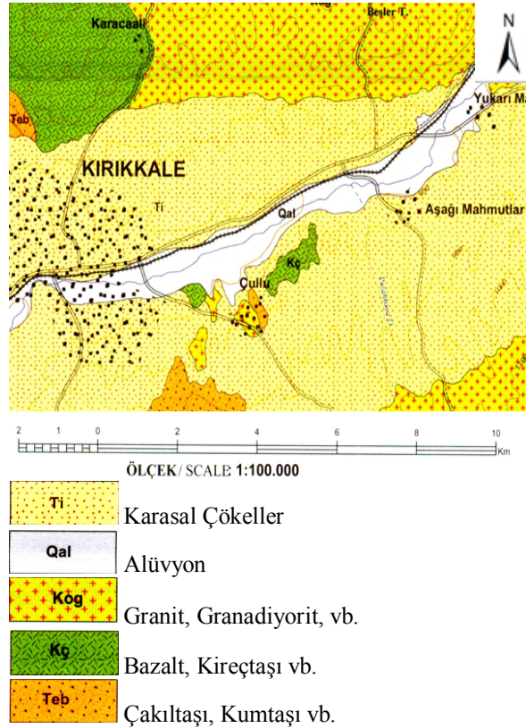
Şekil 2. Kırıkkale ve yakın civarının jeoloji haritası (Geological map of Kırıkkale and its close vicinity) [11]
